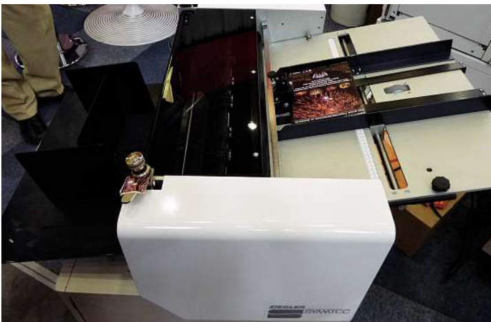
Die neue rotative Rillmaschine PNZ 530 von Ziegler-Symatec verarbeitet bis zu 20.000 Exemplare/h.
